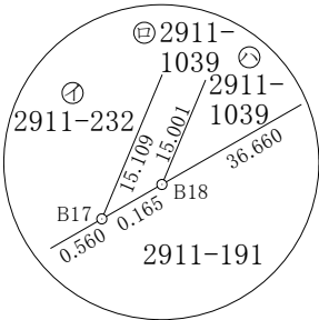
拡大図C
