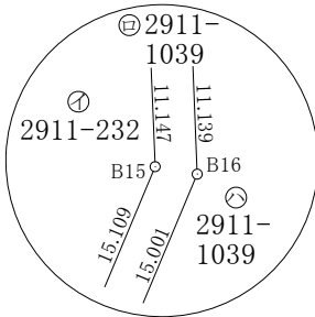
拡大図B
