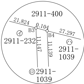
拡大図A
